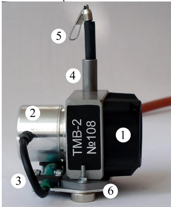
Рис. 3. Датчик перемещения.
