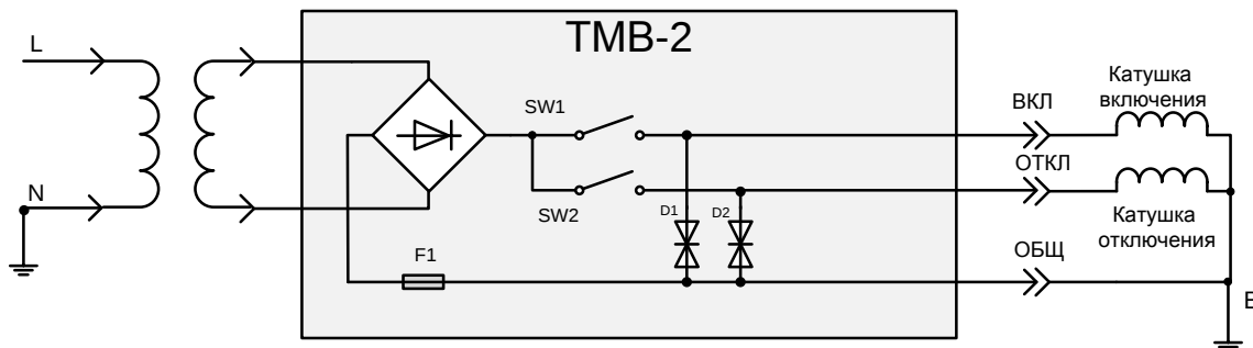
Рис. 20 Применение трансформатора для устранения короткого замыкания при наличии заземления общей шины катушек включения и отключения.
