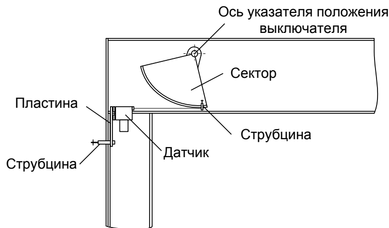
Рис. 6. Установка датчика на выключатель типа ВМТ
